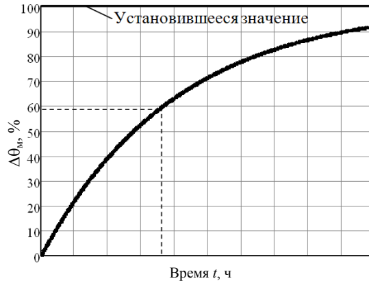
Рис. 1. Экспоненциальная кривая нагрева трансформатора
