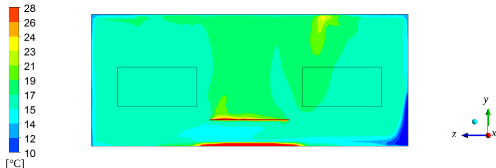
Рис. 7. Поле температуры в плоскости симметрии цеха ( z – y )
