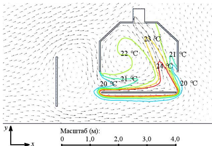
Рис. 6. Поля температуры и скорости при наличии бокового потока воздуха и экрана
