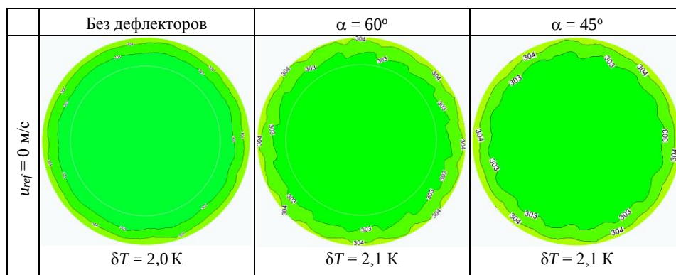
Рис. 5. Поля температуры газовой фазы в горизонтальном сечении БИГ ( h = 30 \text{ м} ) при различных скоростях ветра, конфигурация «в» (см. окончание на с. 55)
