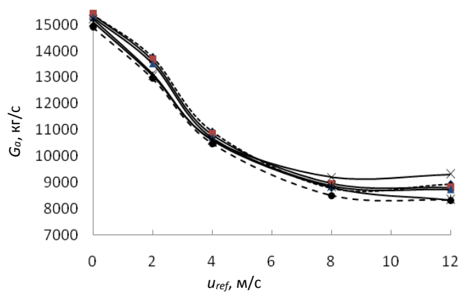
Рис. 6. Полный массовый расход воздуха в градирне (кг/с) как функция скорости ветра, конфигурация системы «б»: ---♦--- — без дефлекторов; —■— — \alpha = 90^\circ ; —▲— — \alpha = 70^\circ ; —×— — \alpha = 60^\circ ; —*— — \alpha = 52^\circ ; ---●--- — \alpha = 45^\circ
