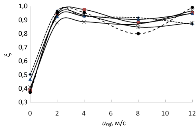
Рис. 8. Параметр неоднородности скорости на выходе из БИГ как функция скорости ветра, конфигурация «б» (обозначения такие же, как на рис. 6)
