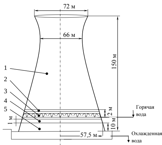
Рис. 1. Схема башенной испарительной градирни: 1 – надоросительное пространство; 2 – каплеуловитель; 3 – разбрызгиватель; 4 – ороситель; 5 – зона дождя; 6 – бассейн
