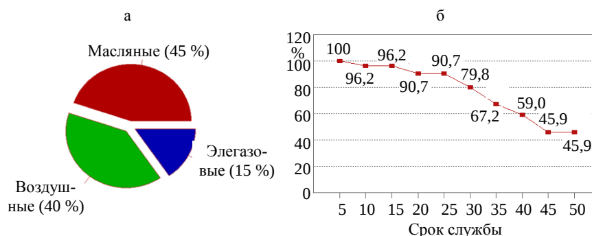
Рис. 9. Изменение относительного числа выключателей: а – по виду дугогасительной среды; б – в зависимости от срока службы
