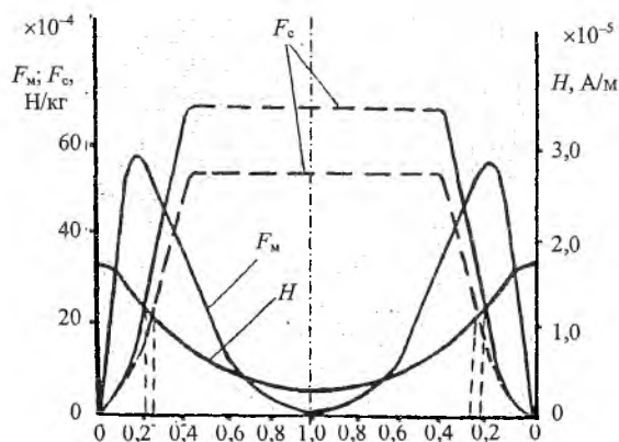
Рис. 1. Эпюры сил, действующих в поровом канале высокоградиентной среды при H_0 = 150 кА/м, \mu = 10,6 : — — — при n = 1 , k = 0,001 Гц/м 2 ; — при n = 0,952 , k = 0,004 Гц/м 2 ( k — коэффициент консистенции)
