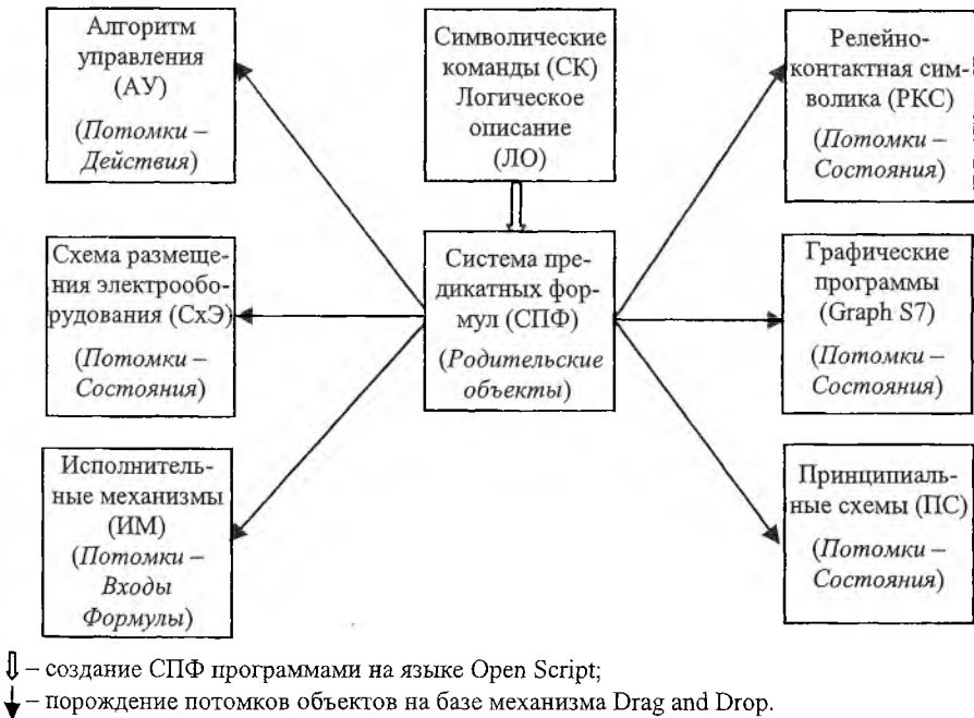
Рис. 2. Концептуальная схема построения распределенной модели
