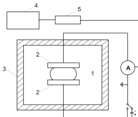
Рис. 3. Схема установки для электризации образцов: 1 – образец; 2 – электроды; 3 – термостат; 4 – регулятор температуры; 5 – двухкоординатный самописец
