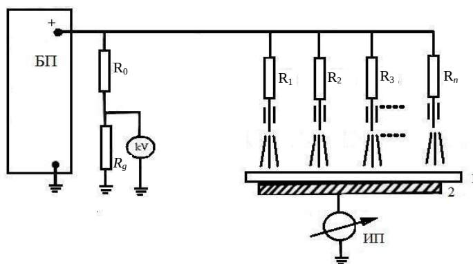
Рис. 1. Принципиальная электрическая схема: БП – блок питания; кV – киловольтметр; R_0 , R_g – омический делитель; R_1 , R_2 , ..., R_n – ограничивающие резисторы; ИП – измерительный прибор; 1 – металлическая подложка; 2 – электрод
