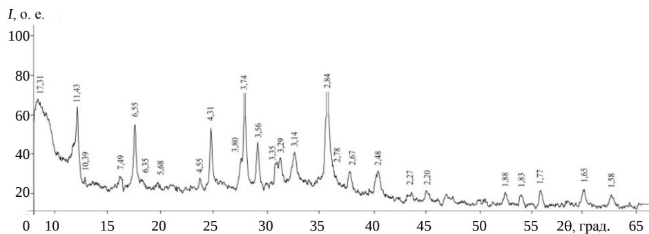
Рис. 6. Рентгенодифрактограмма образца однофазного цеолита, обработанного электрическим разрядом
