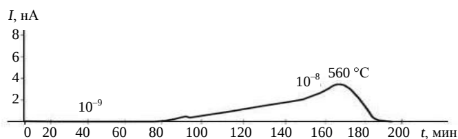
Рис. 4. Кривая термостимулированного тока
