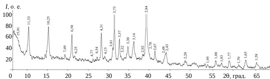
Рис. 5. Рентгенодифрактограмма образца однофазного цеолита, не обработанного электрическим разрядом
