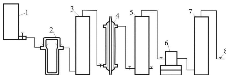
Рис.2. Схема технологической установки для очистки сточных вод: 1 – объем для воды; 2 – реометр; 3 – отстойник; 4 – озонатор; 5 – цеолитовая колонка; 6 – насос; 7 – отстойник; 8 – вентиль
