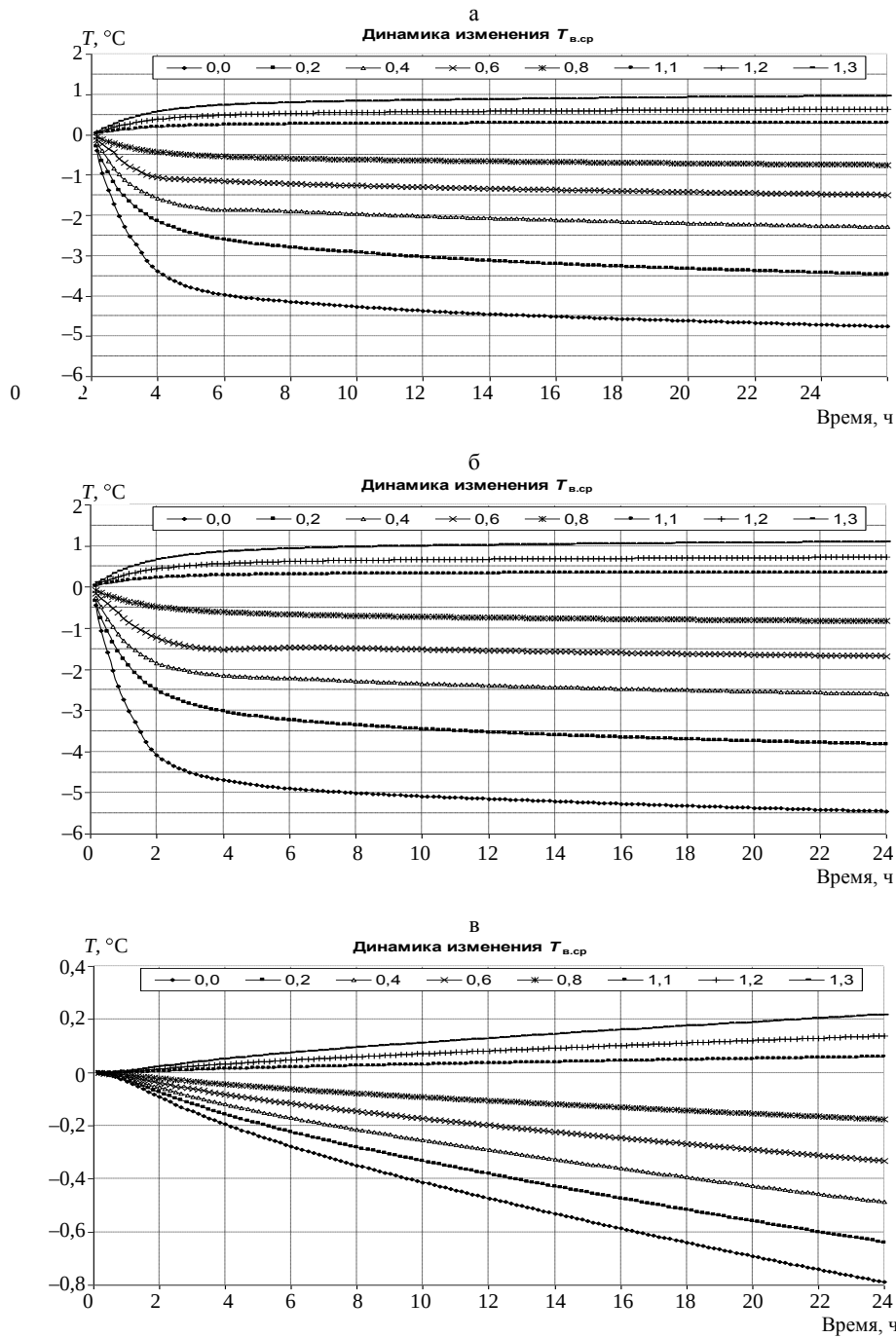
Рис. 3. Графики изменения T_{в.ср} для T_n = 8 ^\circ\text{C} ( Q_{tot} = 80 \text{ Вт} ): а – радиатор; б – конвектор; в – напольное отопление
