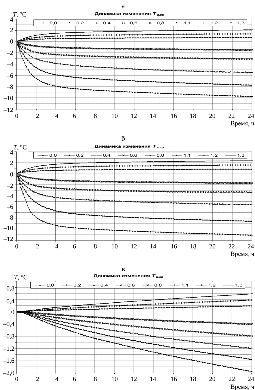
Рис. 2. Графики изменения T_{в.ср} для T_n = -24 ^\circ\text{C} ( Q_{tot} = 190 \text{ Вт} ): а – радиатор; б – конвектор; в – напольное отопление
