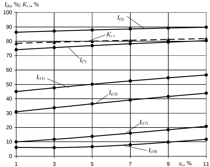
Рис. 5. Зависимости гармонического состава входного тока системы ПЧ–АД от емкости фильтра контура выпрямленного тока C , выраженной величиной \varepsilon_c : S_{Tp} = 1000 \text{ кВ} \cdot \text{А} ; P_{н.АД} = 15 \text{ кВт} , K_n = 100 \%
