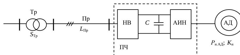
Рис. 1. Схема проведения исследований: Тр – питающий трансформатор; S_{Тр} – номинальная мощность питающего трансформатора; Пр – питающий проводник; L_{Пр} – длина питающего проводника; ПЧ – преобразователь частоты, в состав которого входят: НВ – неуправляемый выпрямитель; С – емкостный фильтр контура выпрямленного тока; АИН – автономный инвертор напряжения; АД – асинхронный двигатель; P_{н.АД} – номинальная мощность АД; K_n – коэффициент нагрузки АД
