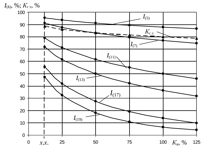
Рис. 4. Зависимости гармонического состава входного тока системы ПЧ–АД от коэффициента нагрузки АД K_n : S_{Tp} = 1000 \text{ кВ} \cdot \text{А} ; P_{н.АД} = 15 \text{ кВт} ; \varepsilon_c = 5 \%
