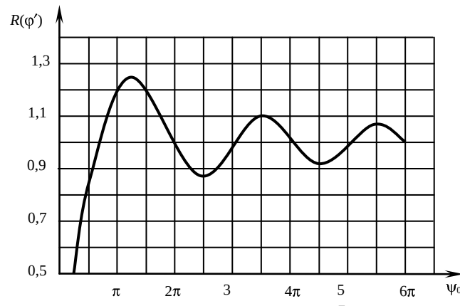
Рис. 2. Зависимость функции R(\phi') от угла пролета \psi_0 электронов между сетками резонатора
