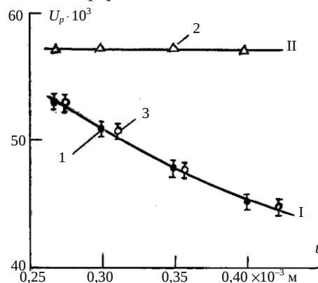
Рис. 4. Разрядное напряжение воздуха между плоскими электродами в зависимости от высоты выступа t на поверхности электрода
