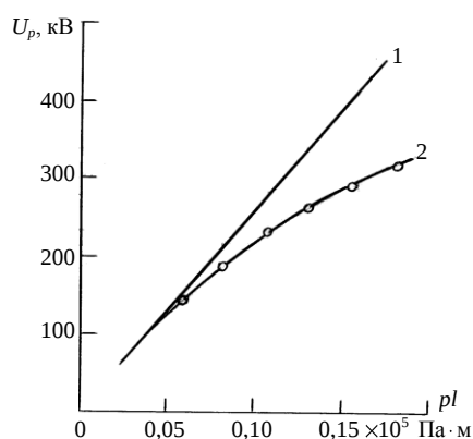
Рис. 1. Зависимости разрядного напряжения воздуха между плоскими электродами от произведения давления p и межэлектродного расстояния l
