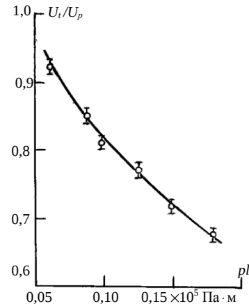
Рис. 3. Относительные значения разрядного напряжения воздуха между плоскими электродами в зависимости от pl
