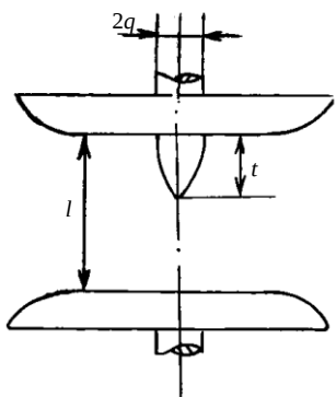
Рис. 2. Плоские электроды с закругленными краями с полуэллипсоидальным выступом
