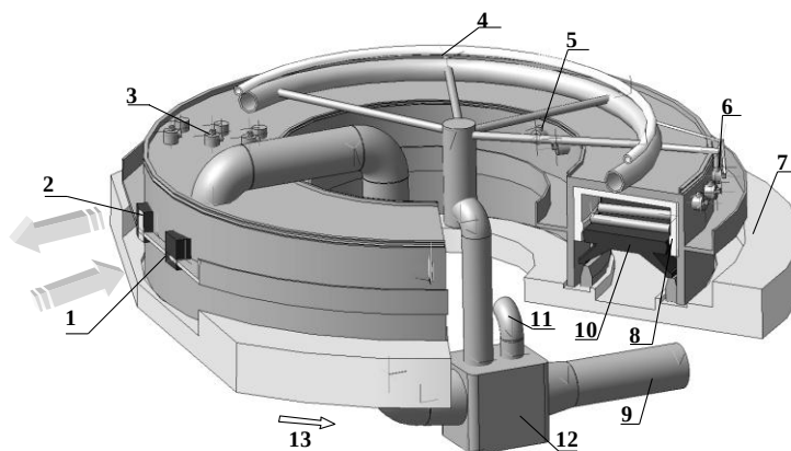
Рис. 1. Общий вид современной кольцевой печи: 1 – окно загрузки; 2 – то же выгрузки; 3 – сводовые плоскопламенные горелки; 4 – газо- и воздухопроводы; 5 – боковые горелки внутреннего кольца; 6 – то же внешнего кольца; 7 – фундамент; 8 – футеровка печи; 9 – дымоотводящий тракт; 10 – подвижный кольцевой под; 11 – вентиляторный воздух к recuperatorу; 12 – recuperator; 13 – направление вращения пода
