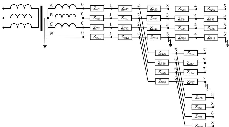
Рис. 2. Схема замещения распределительной линии 0,38 кВ
