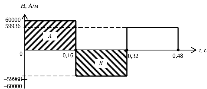
Рис. 2. Зависимость интенсивности спада размагничивающего поля от времени
