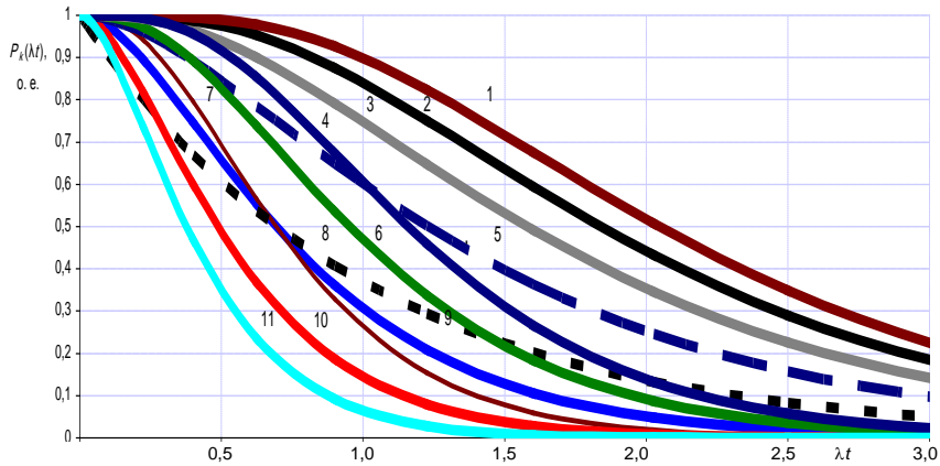
Рис. 1. Вероятности безотказной работы: 1 – k = 4/1 ; 2 – 3/1 ; 3 – 2/1 ; 4 – 1/1 ; 5 – 3/2 ; 6 – 2/2 ; 7 – 0/1 ; 8 – 1/2 ; 9 – 2/3 ; 10 – 1/3 ; 11 – k = 1/4
