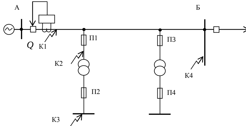
Рис. 1. Схема распределительной сети
