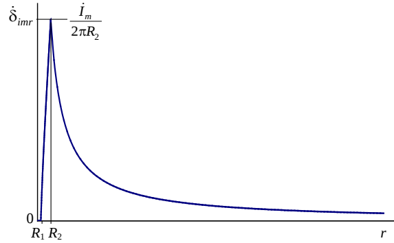
Рис. 2. Зависимость тока \dot{\sigma}_{imr} от координаты r
