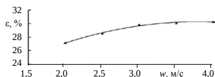
Рис. 6. Влияние лопастного раскручивателя на степень снижения сопротивления циклона при различной скорости газа в нем
