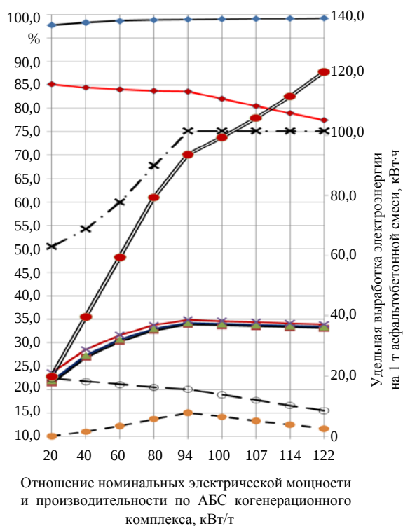
Рис. 3. Влияние электрической мощности когенерационного комплекса, обеспечивающего тепловые нагрузки подготовительного производства АБЗ, на его относительные эксергетические характеристики и удельную выработку электроэнергии: —◆— степень технологического совершенства; —■— степень полного совершенства; —▲— термодинамический КПД; —×— степень термодинамического совершенства; —●— коэффициент использования топлива; —○— термодинамический КПД сушильно-нагревательного барабана (правая ось); —□— термодинамический КПД зоны сушки и нагрева; —×— степень термодинамического совершенства генерации СА; —◆— удельная выработка электроэнергии на 1 т асфальтобетонной смеси
