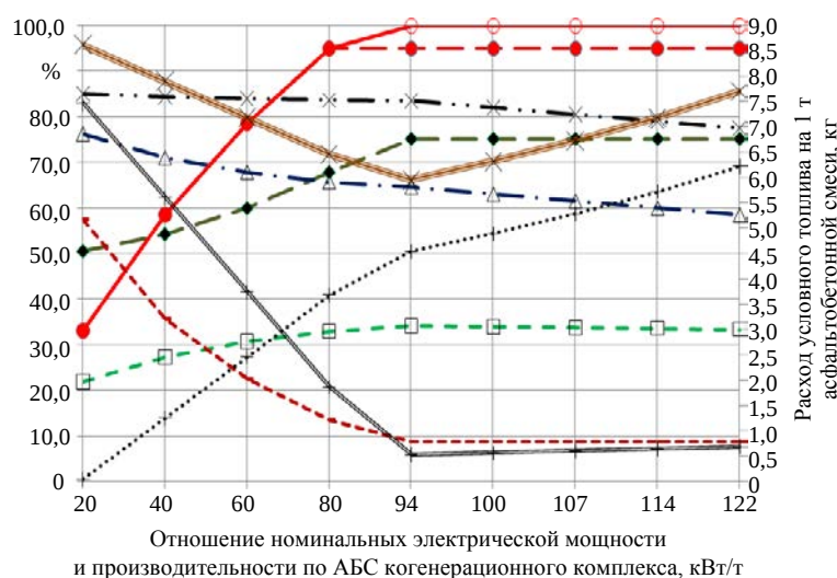
Рис. 2. Влияние электрической мощности когенерационного комплекса, обеспечивающего тепловые нагрузки подготовительного производства АБЗ, на его относительные энергетические характеристики: ◆ — степень термодинамического совершенства генерации СА; □ — термодинамический КПД когенерационного комплекса; △ — энергетический КПД когенерационного комплекса в варианте без использования энергии воды систем охлаждения ДВС; × — энергетический КПД когенерационного комплекса (коэффициент использования топлива); ● — коэффициент теплофикации при сохранении производительности АБЗ; ○ — то же при возможности снижения производительности АБЗ; — — — — процент топлива прямого сжигания в топке СНБ в общем расходе ПГ на когенерационный комплекс; — — — — удельный расход топлива на 1 т АБЗ при расходе топлива на генерацию электроэнергии 318 г/(кВт·ч); × — то же 260 г/(кВт·ч); + — тепловая энергия сетевой воды в 1 кг у. т. на 1 т АБЗ
