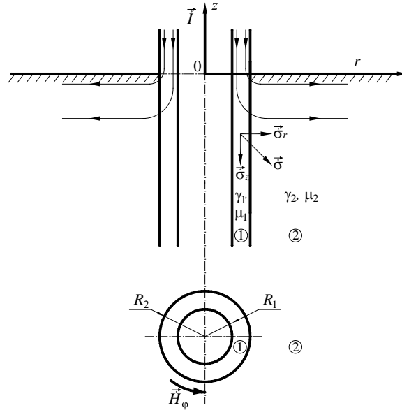
Рис. 1. Геометрическая модель уединенного бесконечно длинного стержневого заземлителя
