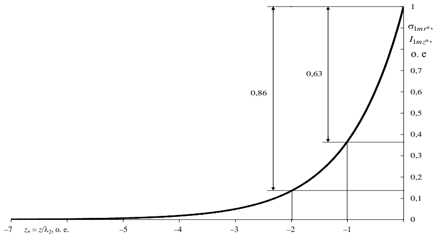
Рис. 2. Распределение радиальной составляющей плотности тока на боковой поверхности заземлителя \sigma_{1mr^*} = \sigma_{2mr^*} = |\dot{\sigma}_{1mr}(R_2, z)|/|\dot{\sigma}_{1mr}(R_2, 0)| и вертикального тока в заземлителе
