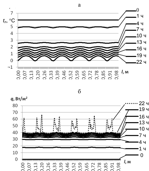
Рис. 4. Температурное поле (а) и тепловой поток (б) на поверхности охлаждаемой воды в разные моменты времени от начала намораживания ледового поля (I и II этапы)
