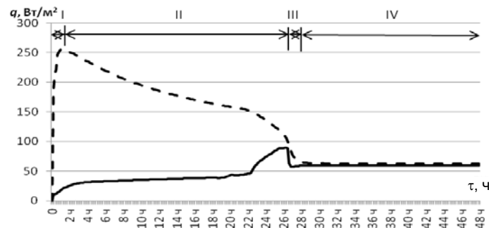
Рис. 3. Изменение теплового потока на поверхности воды и плиты охлаждения при намораживании ледового поля: — — среднее значение теплового потока на поверхности воды (льда); - - - - то же на поверхности плиты охлаждения
