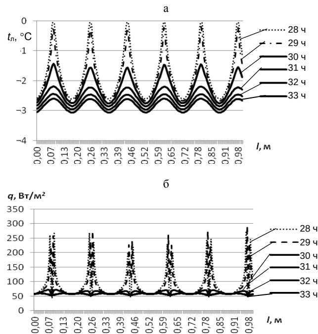
Рис. 6. Температурное поле (а) и тепловой поток (б) на поверхности охлаждаемой воды в разные моменты времени от начала намораживания ледового поля (II, III и IV этапы)
