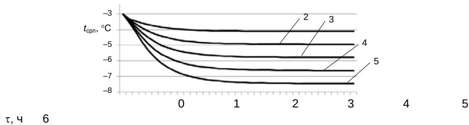
Рис. 8. Изменение средней температуры поверхности льда ( t_{срл} , °C) с течением времени ( \tau , ч) при понижении температур хладагителя ( t_{хп}/t_{х0} , °C): 1 – t_{хп}/t_{х0} = (-8/-5) °C; 2 – (-9/-6) °C; 3 – (-10/-7) °C; 4 – (-11/-8) °C; 5 – t_{хп}/t_{х0} = (-12/-9) °C
