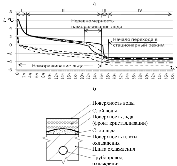
Рис. 2. а – изменение температуры на поверхности воды и плиты охлаждения при намораживании ледового поля: — — минимальная (снизу) и максимальная (сверху) температуры на поверхности воды (льда); - - - - минимальная (снизу) и максимальная (сверху) температуры воды (льда) на поверхности плиты охлаждения; — · — — среднее значение температуры воды (льда) ( t_0 = 6 °С; t_{хп} = -7 °С; t_{хп} = -4 °С; t_b = 8 °С; \delta_n = 40 мм); б – фрагмент бетонной плиты охлаждения при намораживании льда
