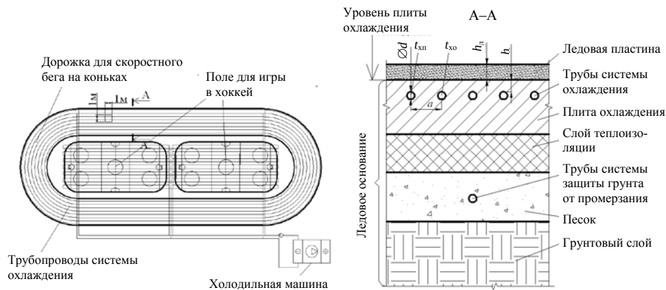
Рис. 1. Система охлаждения ледового поля, разрез А–А основания ледового поля: d – диаметр труб системы охлаждения, мм; a – шаг укладки трубопроводов, мм; h_b – толщина слоя бетона над трубами системы охлаждения, мм; h_l – толщина ледовой пластины, мм; t_{xл} – температура хладоносителя в подающем трубопроводе, °С; t_{xо} – температура хладоносителя в обратном трубопроводе, °С
