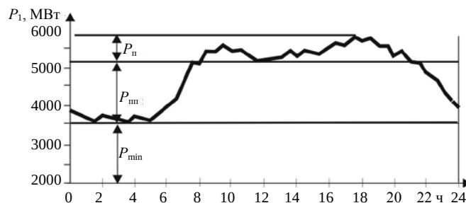
Рис. 4. Типовой суточный график нагрузки энергетической системы Беларуси в 2007 г. в отопительный период: P_{\min} = 3500 МВт; P_{пп.мах} = 1680 МВт; P_{п.мах} = 660 МВт
