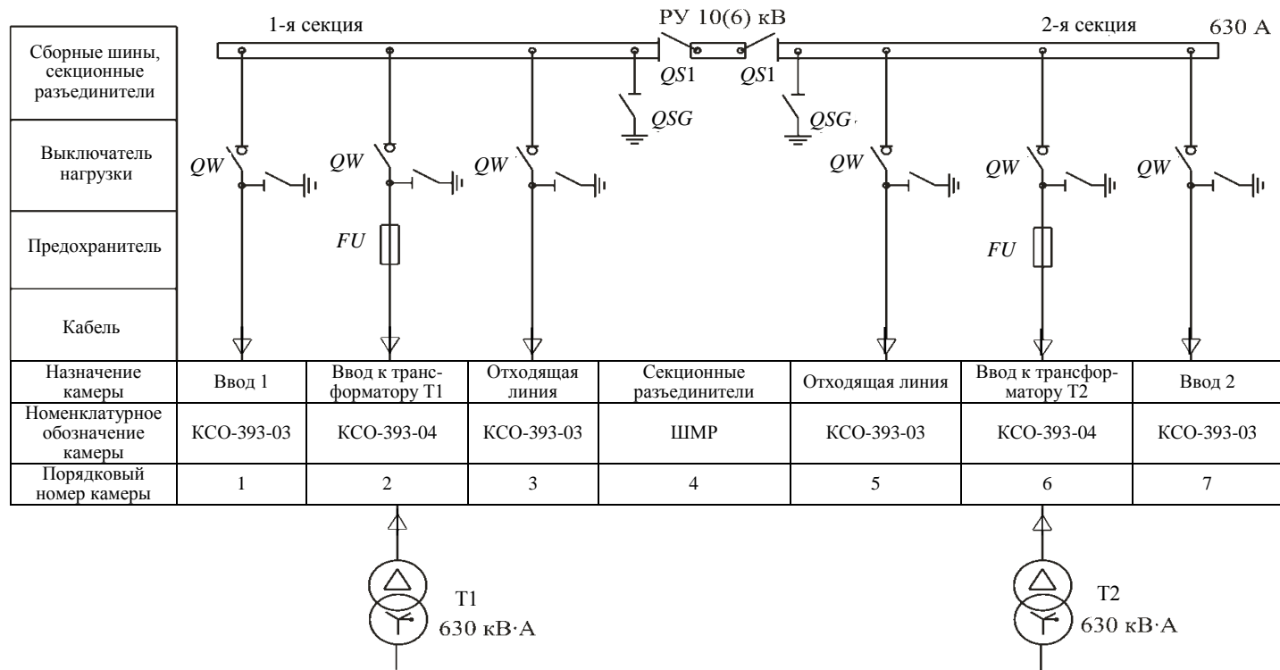
Рис. 3. Схема электрических соединений РУ 6–10 кВ ТП, выполненного камерами типа КСО (вариант 1)
