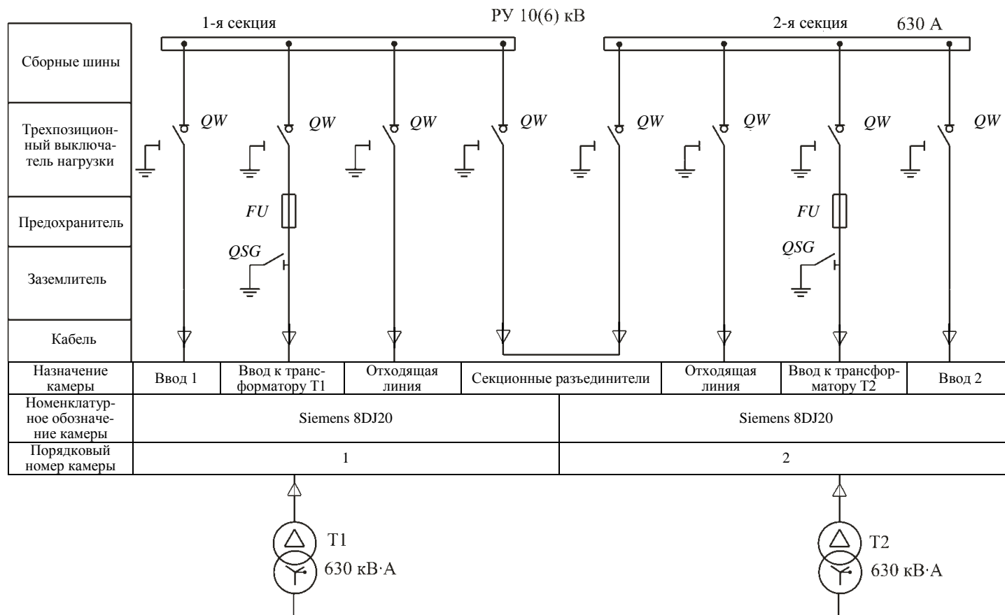
Рис. 4. Схема электрических соединений РУ 6–10 кВ ТП, выполненного с использованием КРУЭ (вариант 2)
