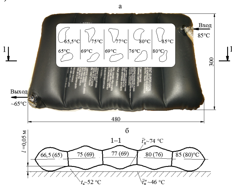
Рис. 1. Общий вид отопительного прибора (а) и расчетная схема (б): l – характерный размер; t'_n , t''_n – соответственно температуры теплоотдающей и тепловоспринимающей поверхностей
