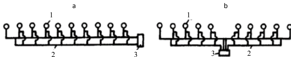
Рис. 1. Типовые схемы скважинных водозаборов с парными сборными водоводами:
