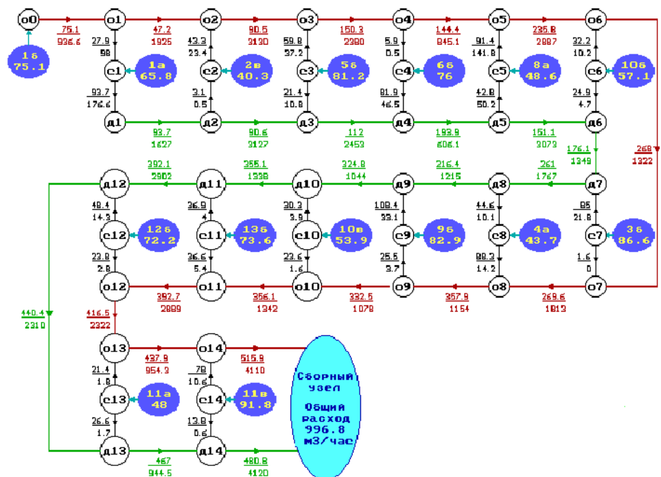
Рис. 4. Пример расчета водозабора с парными сборными водоводами согласно указанному алгоритму
