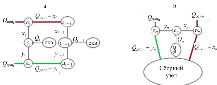
Рис. 3. Схемы для расчета колец парного сборного водозабора:
