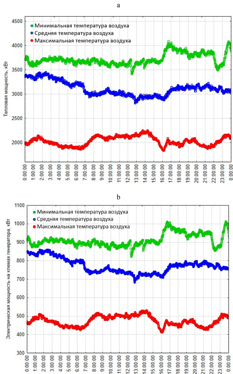
Рис. 4. Суточный график выработки энергии на ORC-установке:
