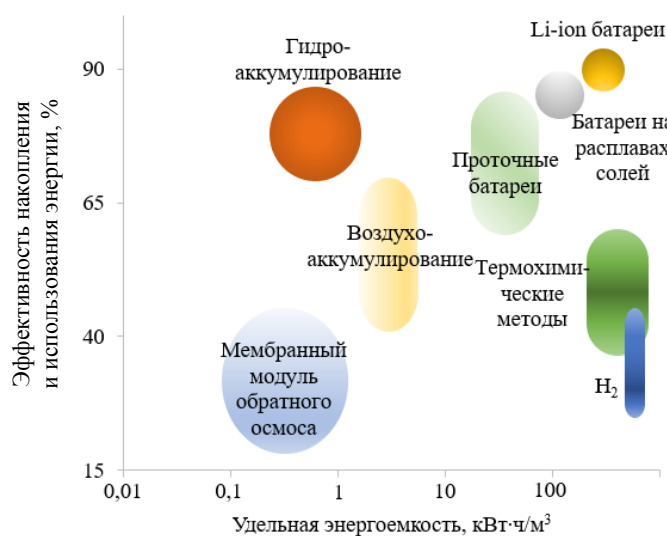
Рис. 1. Зависимость эффективности накопления и использования энергии от удельной энергоёмкости для различных технологий хранения электрической энергии
