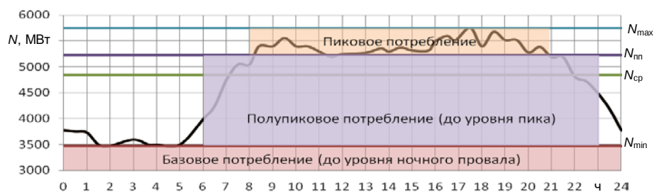
Рис. 1. Типовой суточный график нагрузки ОЭС [4, 5]
