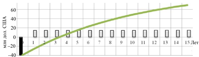
Рис. 4. Изменение денежного потока за период эксплуатации комплексов в варианте зарядки аккумуляторов до 120 °С при ставке дисконтирования 10 %: ■ – капиталовложения; □ – прибыль; — чистый дисконтированный доход
