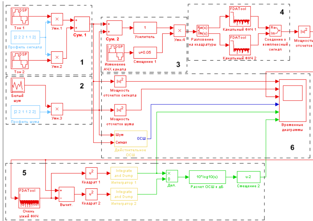
Рис. 1. Модель Simulink алгоритма измерения ОСШ
