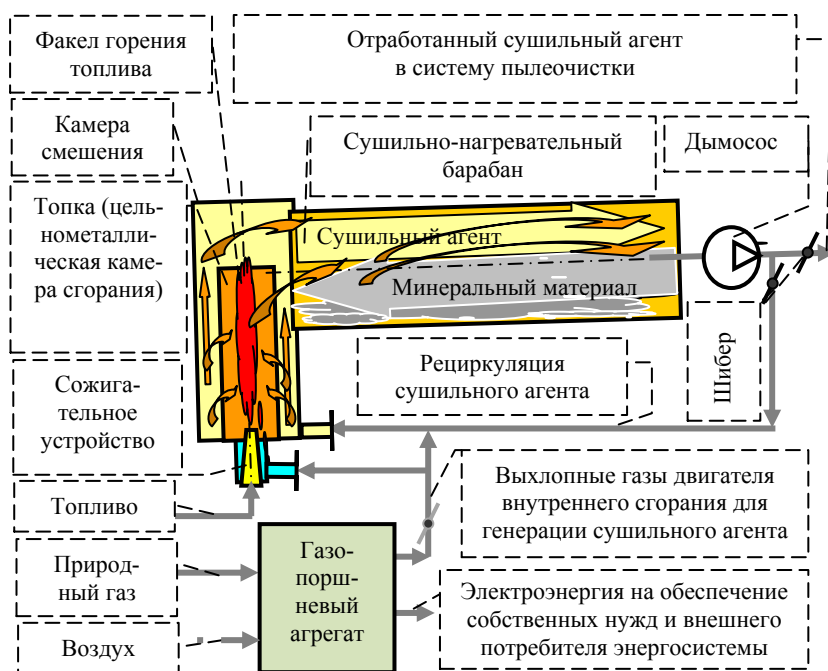
Рис. 1. Схема комплекса для комбинированной выработки энергопоточков на базе теплотехнологии горячей асфальтобетонной смеси, образованная в результате сопряжения ДВС и СНБ
