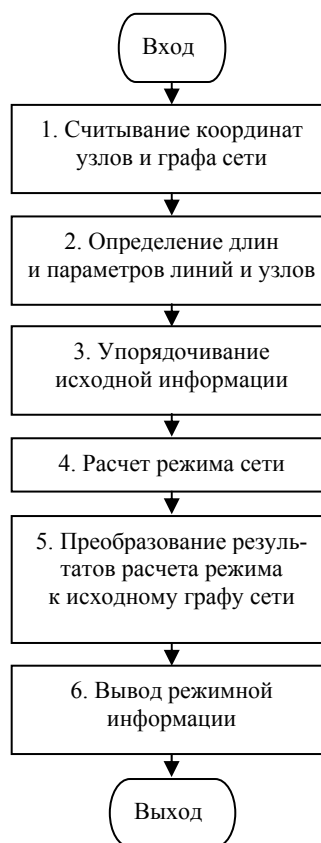
Рис. 4. Схема структурного алгоритма программы
