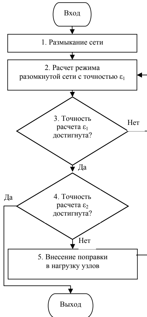
Рис. 6. Схема алгоритма расчета режима
