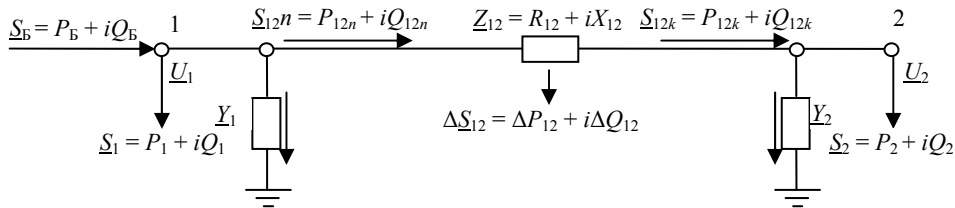
Рис. 5. Схема замещения участка сети
