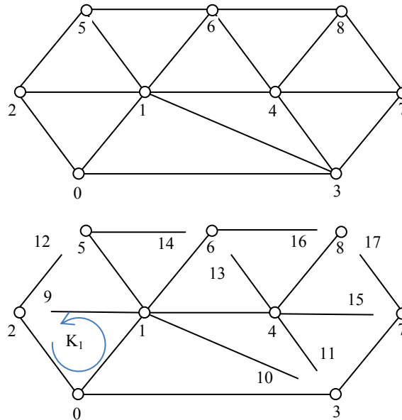
Рис. 7. Преобразование замкнутой сети в разомкнутую
