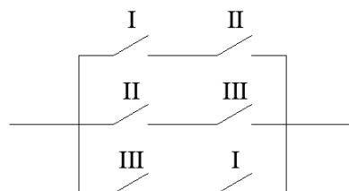
Рис. 3. Мажоритарная схема соединения контактов «два из трех»
