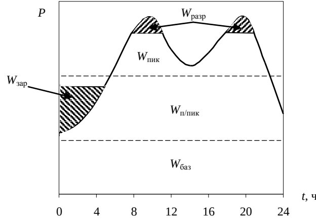
Рис. 1. Применение накопителей электроэнергии для выравнивания суточного графика работы энергосистемы
