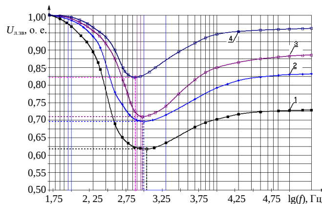
Рис. 2. Зависимость нормированного напряжения на ЛЛ с соизмеримыми значениями междуэлектродных расстояний ( l_{\text{эл}} ), но разными диаметрами колб: 1 – ЛБ 20, l_{\text{эл}} = 50,5 см, P = 20 Вт, d_{\text{тр}} = 38 мм; 2 – ТЛД 18, l_{\text{эл}} = 51 см, P = 18 Вт, d_{\text{тр}} = 26 мм; 3 – ТЛД 14, l_{\text{эл}} = 48 см, P = 14 Вт, d_{\text{тр}} = 16 мм; 4 – ТЛД 13, l_{\text{эл}} = 46 см, P = 13 Вт, d_{\text{тр}} = 7 мм
