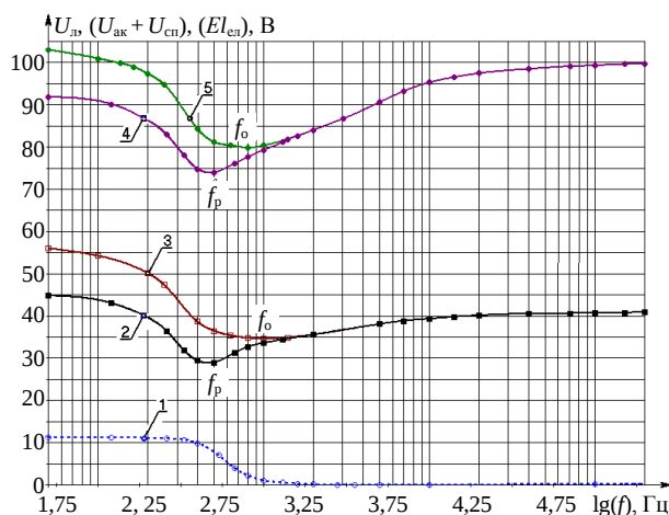
Рис. 3. Зависимости: 1 – суммы анодно-катодного падения потенциала и падения потенциала на отработанных витках спиралей ( U_{\text{ак}} + U_{\text{сп}} ) на СКЛ с l_{\text{эл}} = 4 см; 2, 4 – падение потенциала на положительном столбе разряда ( El_{\text{эл}} ) с минимумом на результирующей частоте f_p ; 3, 5 – напряжений на ЛЛ ( U_{\text{л}} ) ЛБ 20 и ЛБ 40 с минимумом на граничной частоте f_o от частоты напряжения питания соответственно
