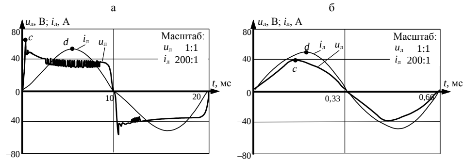
Рис. 6. Осциллограммы токов и напряжений ЛЛ мощностью 8 Вт ( d_{тр} = 16 мм) в цепи с дросселем при номинальном токе лампы и разных частотах напряжения питания: а – 50 Гц; б – 1500 Гц
