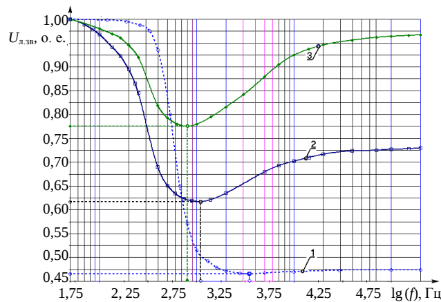
Рис. 1. Зависимость нормированного напряжения на ЛЛ с одинаковым внутренним диаметром колбы ( d_{\text{тр}} = 38 мм), но разными междуэлектродными расстояниями ( l_{\text{эл}} ) (напряжениями): 1 – СКЛ, l_{\text{эл}} = 11,0 см, P = 8 Вт; 2 – ЛБ 20, l_{\text{эл}} = 50,5 см, P = 20 Вт; 3 – ЛБ 40, l_{\text{эл}} = 112,5 см, P = 40 Вт
