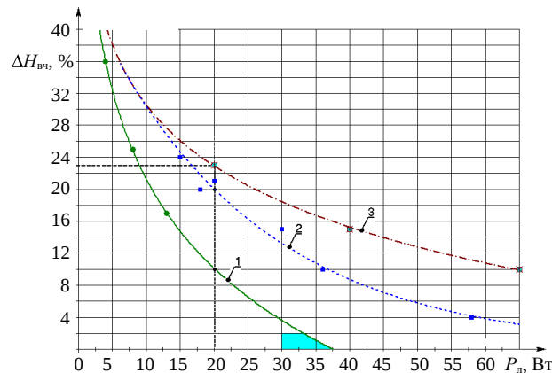
Рис. 7. Зависимость прироста световой отдачи ЛЛ на высоких частотах ( f_m \geq 40 кГц) от мощности (длины) и диаметра колбы: 1 – d_{тр} = 16 мм; 2 – 26 мм; 3 – 38 мм
