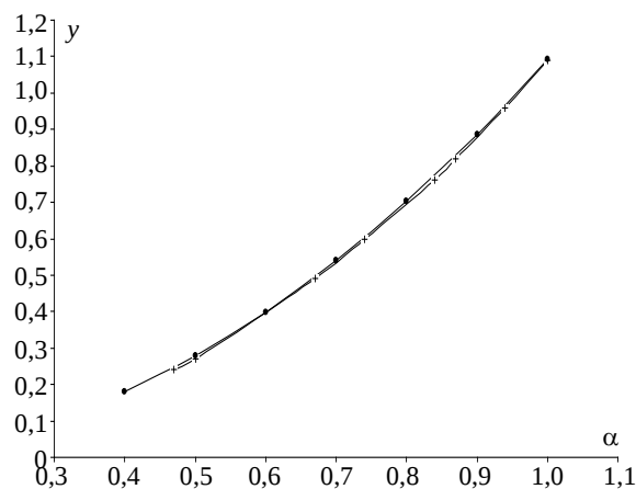
Рис. 1. Зависимость y = f(\alpha) при управлении на постоянство \beta = \text{const} :
